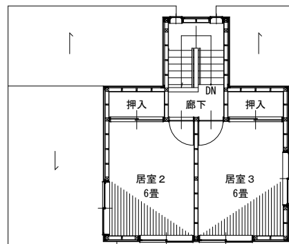
2階平面図
