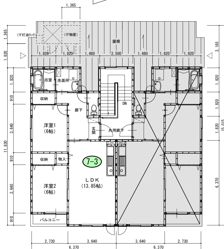
7-3号 (2階2LDK) 平面図
