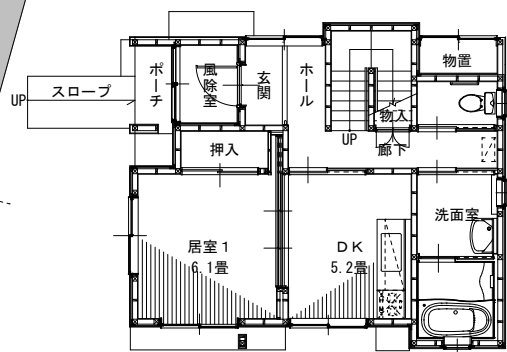
1階平面図
